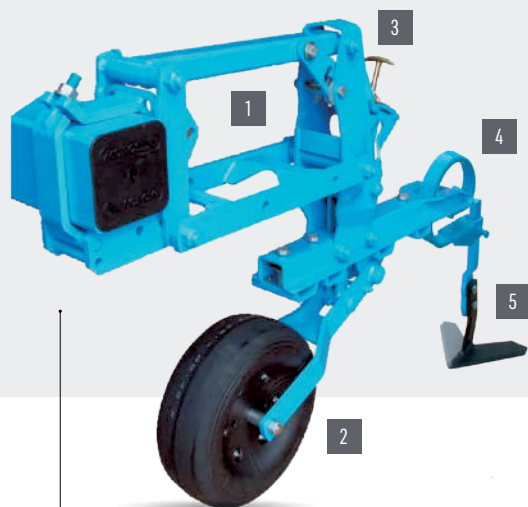
ÉLÉMENT MULTICROP Inter-rang 25 à 90cm
