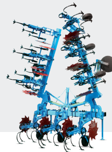
Bineuse TIP 5 pouces à repliage hydraulique 8 rangs à 75cm d'inter-rangs
