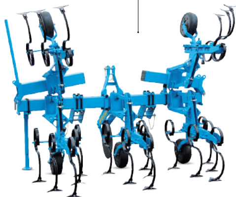
Bineuse TIP 5 pouces à repliage manuel 4 rangs à 75cm d'inter-rang
