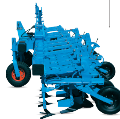
Bineuse frontale «éléments inversés» 12 rangs à 45cm d'inter-rang
